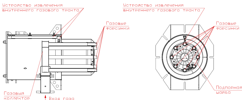
Рис.10 Внутренняя газовая линия горелки Т-5.820 G
