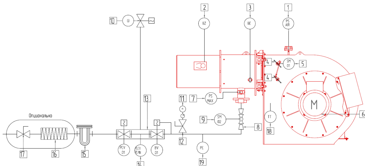
Рис.4. P&ID диаграмма горелки T-5.820 G.E
