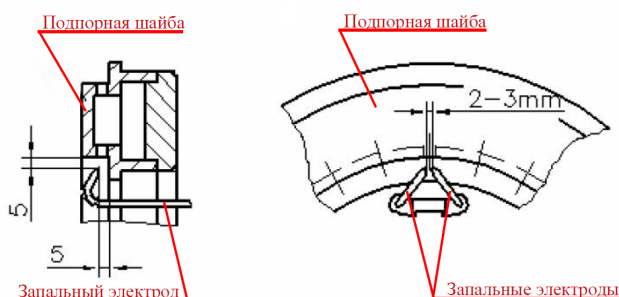
Рис.12 Расположение запальных электродов
