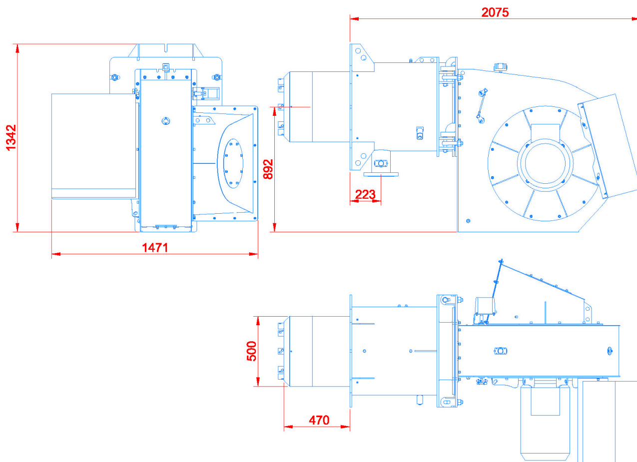
Рис.6 Общий вид горелочного устройства Т-5.820 G.E
