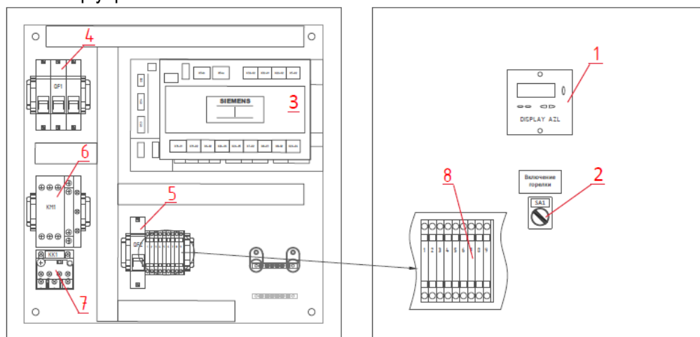
Рис.5. Внешний и внутренний вид шкафа управления горелкой Т-5.820 G.E
