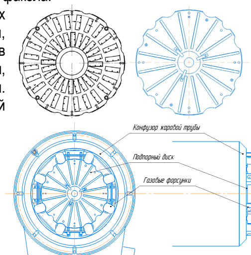
Рис.11 жаровая труба
