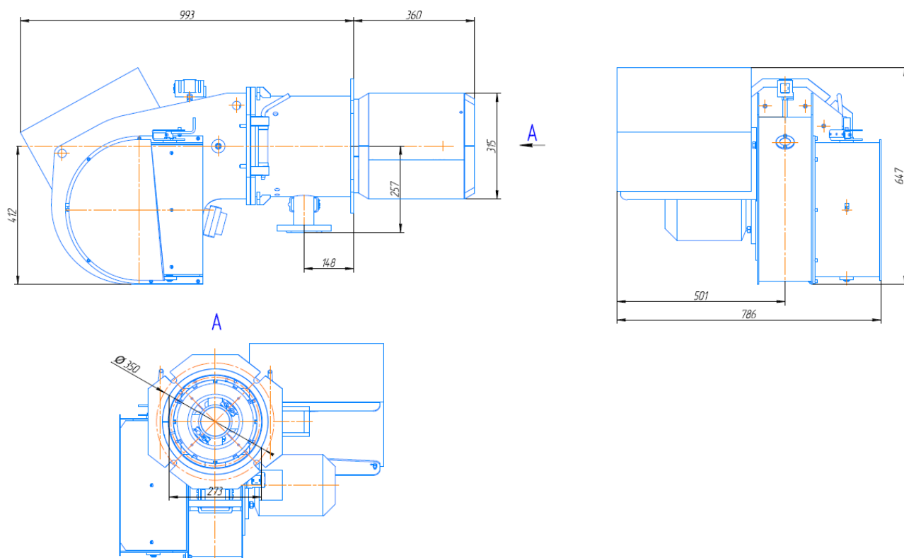
Рис.6 Общий вид горелочного устройства Т-2.165 G.E
