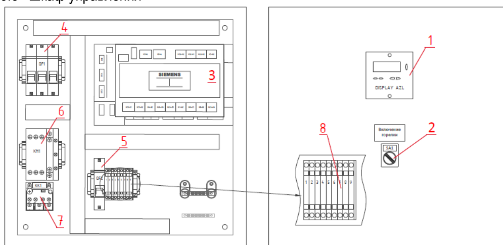
Рис.5. Внешний и внутренний вид шкафа управления горелкой Т-2.165 G.E
