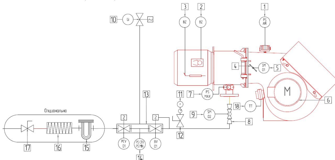
Рис.4. P&ID диаграмма горелки T-2.165 G.E
