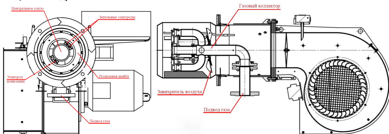
Рис.10 Внутренняя газовая линия горелки T-2.165 G
