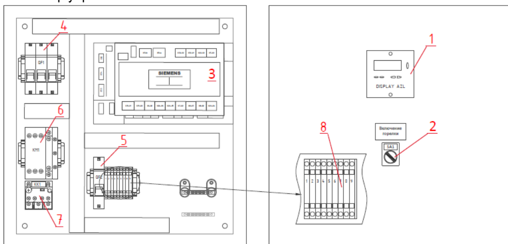
Рис.5. Внешний и внутренний вид шкафа управления горелкой T-5.630 G.E
