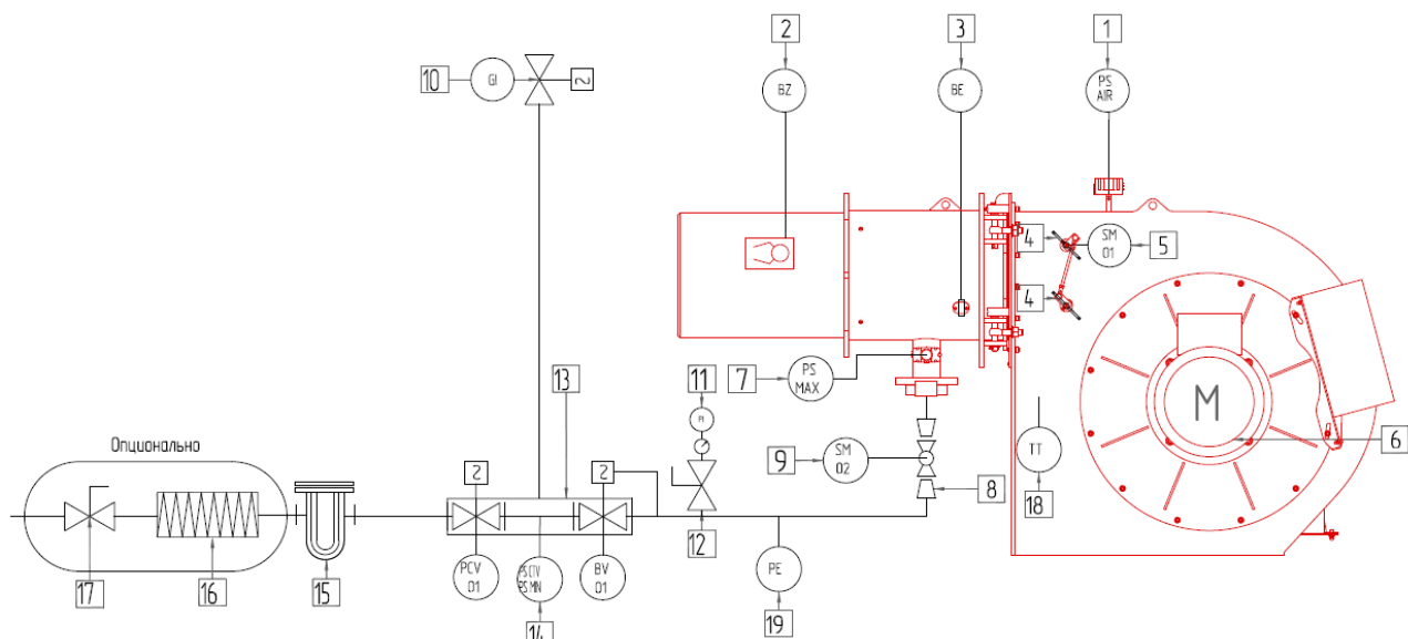
Рис.4. P&ID диаграмма горелки T-5.630 G.E
