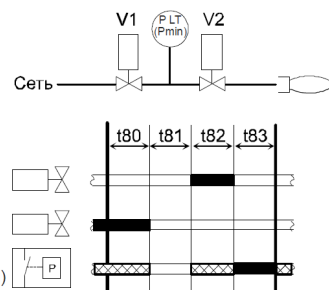
Рис.14 Контроль герметичности
