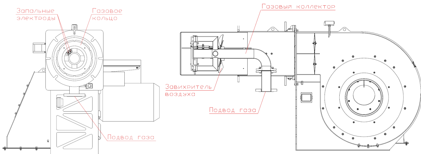
Рис.10 Внутренняя газовая линия горелки Т-5.630 G
