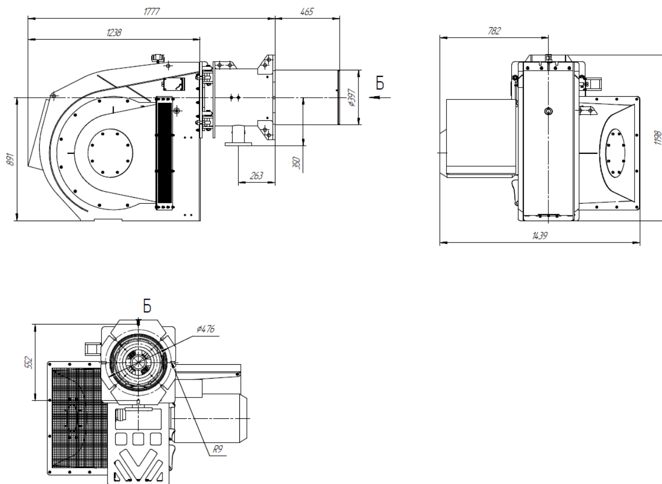
Рис.6 Общий вид горелочного устройства T-5.630 G.E
