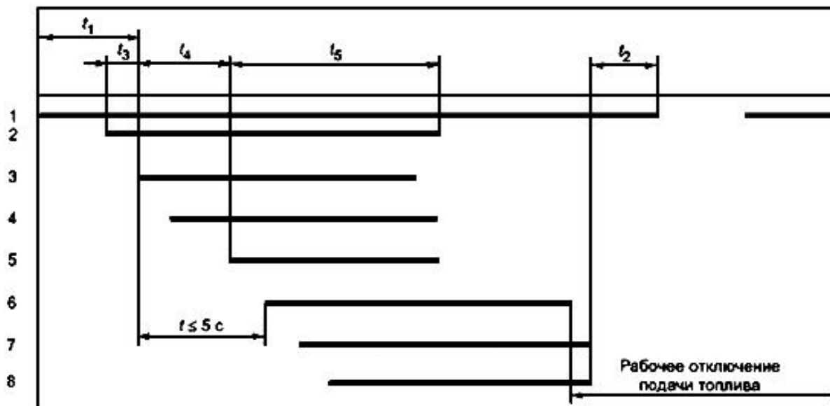
Диаграммы с защитным отключением при пуске
