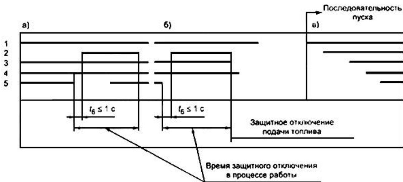
а - с положительным результатом; б - безрезультатно; в - с повторным пуском после вмешательства обслуживающего персонала; 1 - поток воздуха; 2 - запальное устройство; 3 - сигнал подачи топлива; 4 - подача топлива; 5 - наличие пламени
